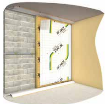
Mise en place des lés de membrane Vario® Xtra
