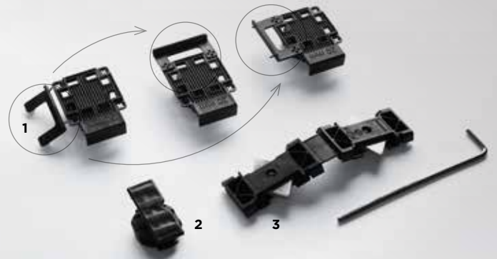
1: clip vertical multi-réglable P 9238 2: clip rotatif horizontal P 9237 3: clip d'angle flexible P 9239
